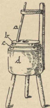
Handmühle aus Schlesien. a) Handtange. b) Laufstein. c) Boden- stein. d) Holzblock.
