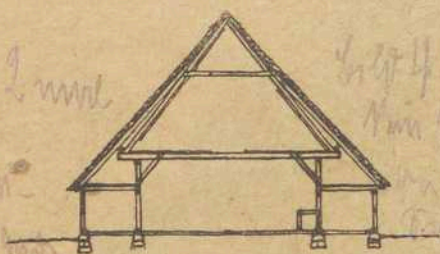
Stizze 3. Querschnitt zu Typ 2.
