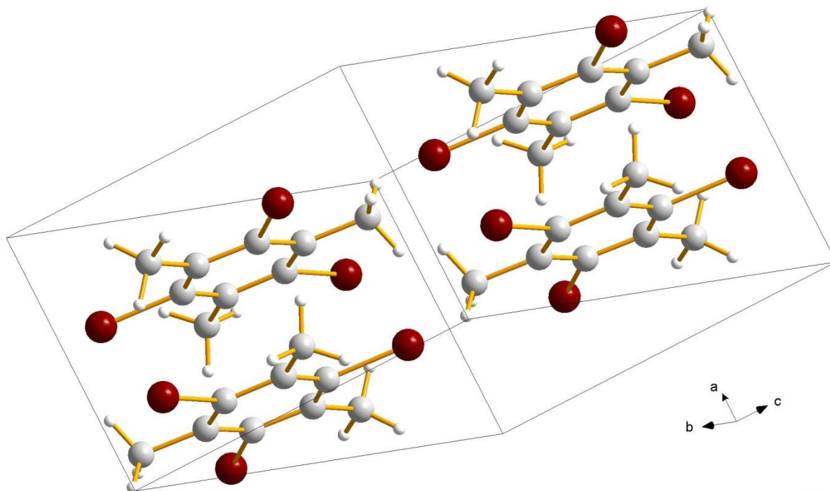
Abbildung 6. Darstellung der Elementarzelle von 1,3,5-Tribrommesitylen. Farbkodierung: H weiß, C grau, Br braun.
