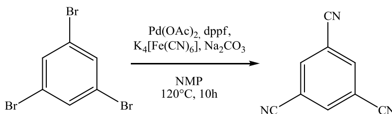
Schema 1. Reaktion von 1,3,5-Tribrombenzen zu 1,3,5-Tricyanobenzen.
