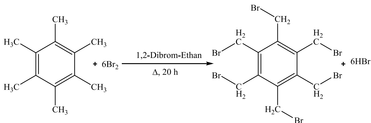
Schema 19. Reaktion von Hexamethylbenzen zu Hexakis(bromomethyl)benzen.
