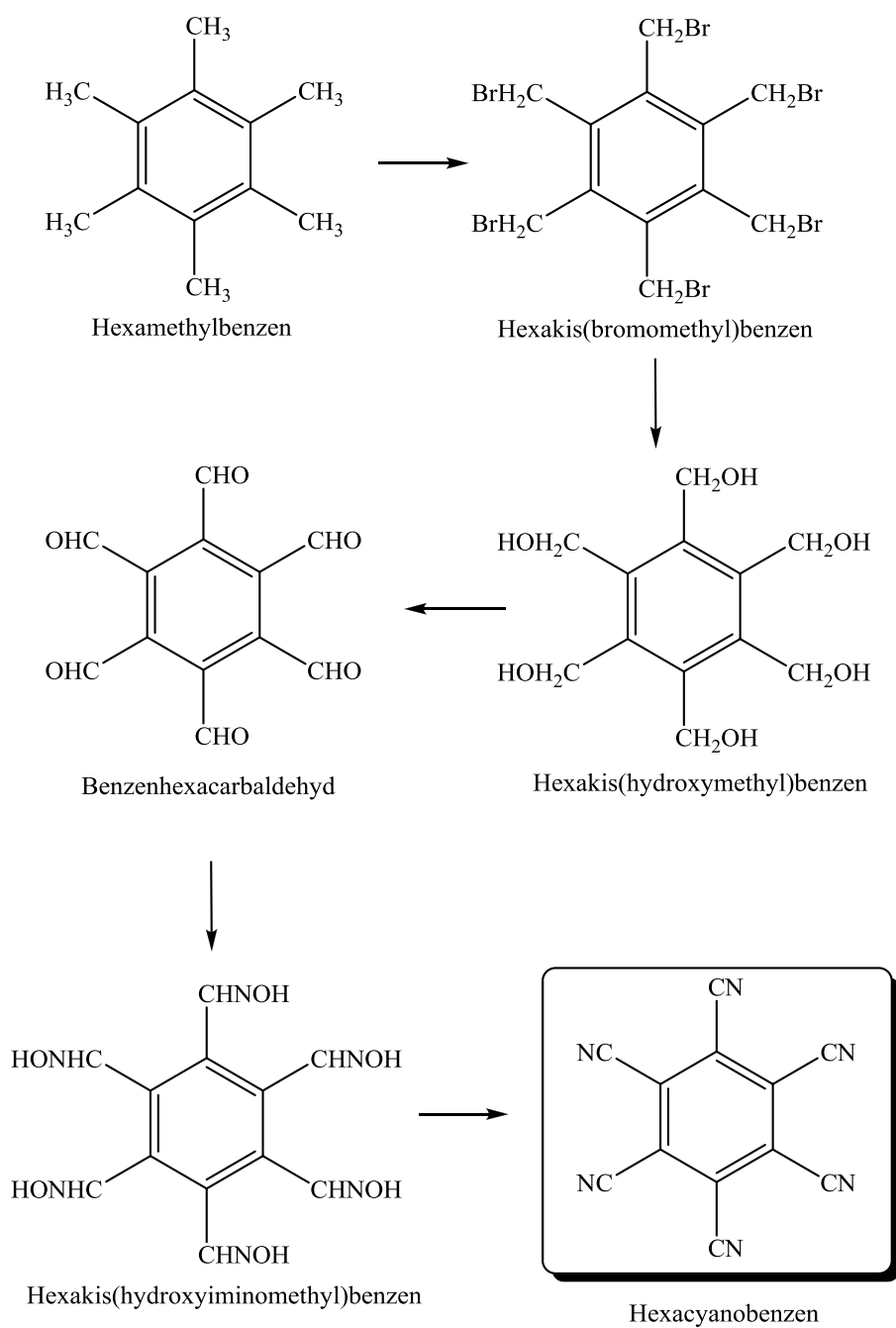
Schema 17. Geplante Syntheseroute zu Hexacyanobenzen.
