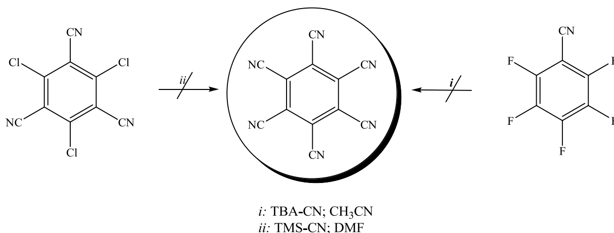
Schema 5. Syntheserversuche des Hexacyanobenzens, TBA-CN – Tetrabutylammoniumcyanid, TMS-CN – Trimethylsilylcyanid.
