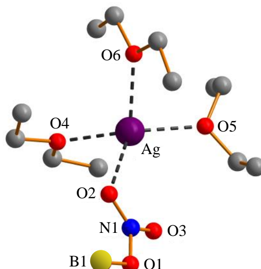
Abbildung 31. Ag + -Koordination im [Ag(Et 2 O) 3 ] + [NO 3 •B(C 6 F 5 ) 3 ]. Ausgewählte Abstände (Å) und Winkel (°): O2–Ag 2.504(3), Ag–O4 2.353(3), Ag–O5 2.313(3), Ag–O6 2.405(3); O4–Ag–O5 138.3(1), O5–Ag–O6 88.8(1), O4–Ag–O6 106.8(1), O2–Ag–O5 117.8(1), O2–Ag–O4 86.6(1), O2–Ag–O6 122.2(1).
