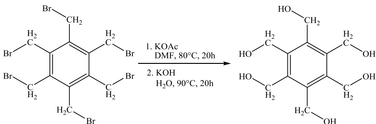
Schema 20. Reaktion von Hexakis(bromomethyl)benzen zu Hexakis(hydroxymethyl)benzen.
