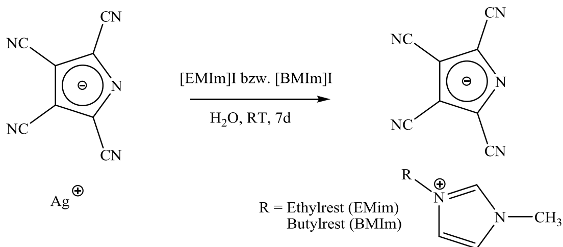
Schema 29. Synthese von 1-Ethyl-3-methylimidazolium- und 1-Butyl-3-methylimidazolium-tetracyanopyrrolid.
