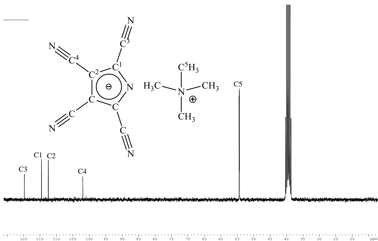
Abbildung 23. ^{13}\text{C} -NMR Spektrum von Tetramethylammonium-tetracyanopyrrolid, DMSO- \text{D}_6 , 75 MHz
