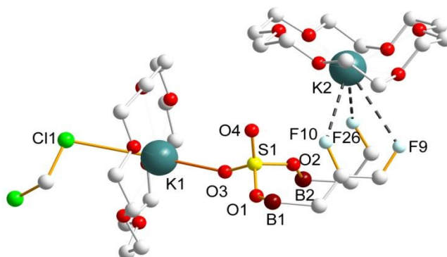
Abbildung 35. K + -Koordination im [K(18-Krone-6)(CH 2 Cl 2 )] 2 + [SO 4 •2 B(C 6 F 5 ) 3 ] 2 - . Wasserstoffatome weggelassen. C 6 F 5 - Gruppe reduziert auf den Teil, der mit K2 über F-Atome koordiniert. Ausgewählte Abstände (Å) und Winkel (°): O3–K1 2.619(2), K1–Cl1 3.339(2), K1–O4 4.388(3), K2–O4 4.079(3), F9–K2 3.486(2), F10–K2 3.096(2), F26–K2 2.758(2), F9–F10 2.033(3), F9–F26 3.162(3), F10–F26 3.301(3); Cl1–K1–O3 156.80(6), F26–K2–F10 68.38(5), F26–K2–F9 59.49(5), F9–K2–F10 46.70(5).
