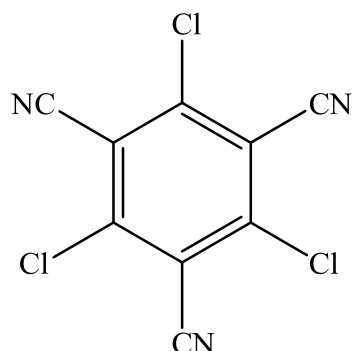
Schema 16. 1,3,5-Trichloro-2,4,6-tricyanobenzen.
