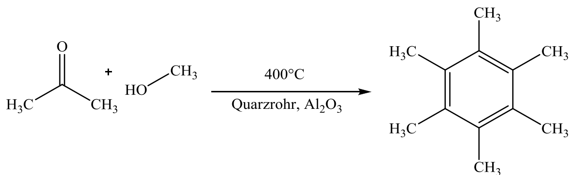
Schema 18. Reaktion von Aceton und Methanol zu Hexamethylbenzen.
