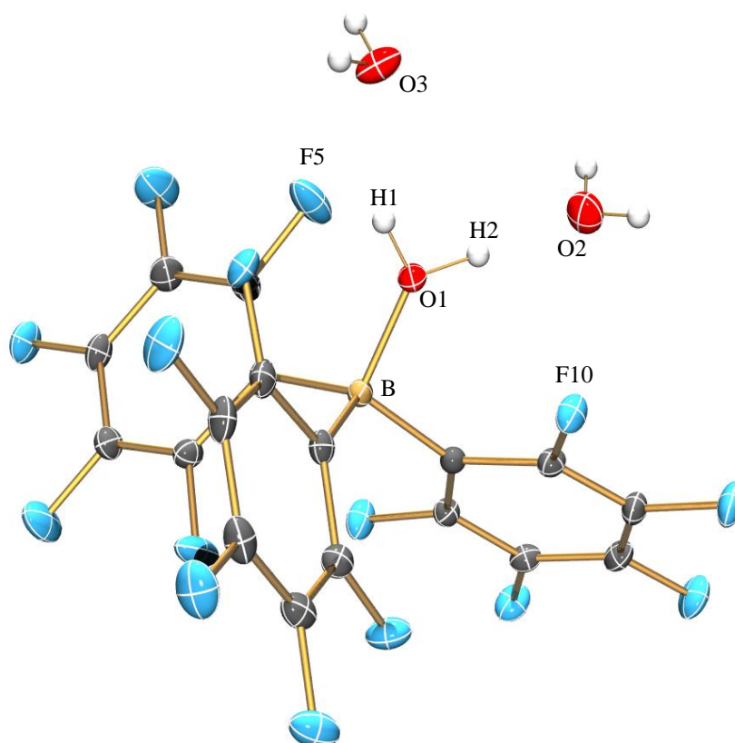
Abbildung 36. ORTEP-Darstellung der Molekülstruktur von B(C_6F_5)_3 \cdot 3H_2O . Thermische Ellipsoide entsprechen 50% Wahrscheinlichkeit bei 173 K. Ausgewählte Abstände (Å) und Winkel (°): O1–B 1.582(2), O1–H1 0.98(3), O1–H2 0.83(2), O2–H3 0.79(3), O2–H4 0.82(3), O3–H5 0.82(3), O3–H6 0.85(3); B–O1–H1 124.2(15), B–O1–H2 126.9(16), H1–O1–H2 107(2), H3–O2–H4 112(3), H5–O3–H6 108(3).
