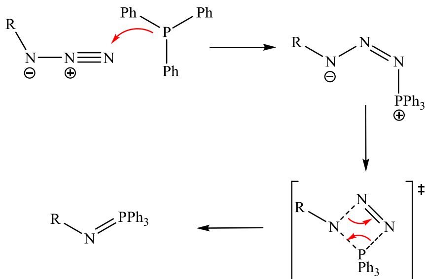
Schema 24. Reaktionsmechanismus der Staudinger-Reaktion.
