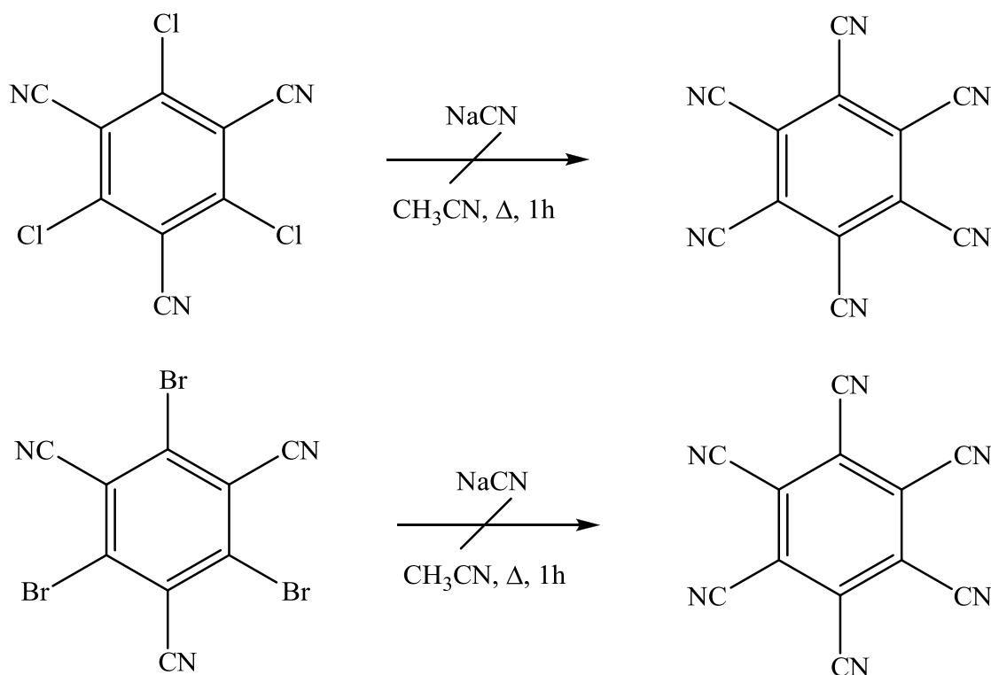
Schema 22. Keine Reaktion von 1,3,5-Trihalogeno-2,4,6-tricyanobenzen zu Hexacyanobenzen.
