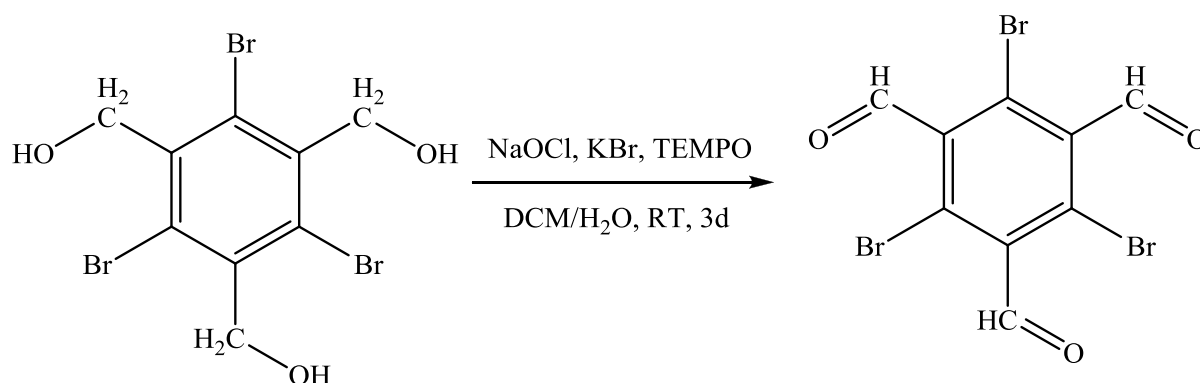
Schema 10. Reaktion von 1,3,5-Tribromo-2,4,6-tris(hydroxymethyl)benzen zu 2,4,6-Tribromo-1,3,5-benzenetricarbaldehyd.
