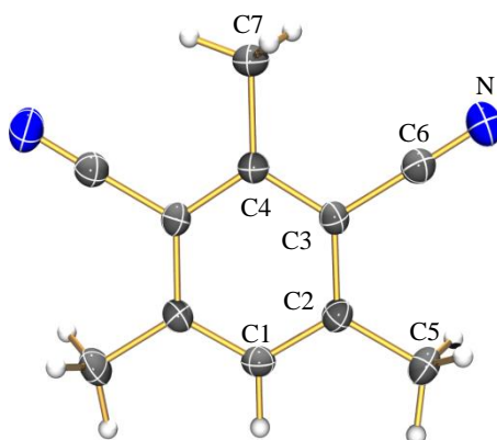
Abbildung 3. ORTEP-Darstellung der Molekülstruktur von 1,3-Dicyanomesitylen. Thermische Ellipsoide entsprechen 50% Wahrscheinlichkeit bei 173 K. Farbkodierung: H weiß, C grau, N blau. Ausgewählte Abstände (Å) und Winkel (°): C2–C1 1.384(1), C2–C5 1.496(2), C3–C4 1.395(1), C3–C2 1.408(2), C3–C6 1.449(2), C4–C3 i 1.395(1), C4–C7 1.506(2), C6–N 1.124(2); C4–C3–C2 122.4(1), C4–C3–C6 118.6(1), C2–C3–C6 119.02(9), C3–C4–C3 i 117.0(1), C3–C4–C7 121.49(7), C3 i –C4–C7 121.49(7), C1–C2–C3 118.1(1), C1–C2–C5 121.1(1), C3–C2–C5 120.8(1), C3–C6–N 179.1(1).
