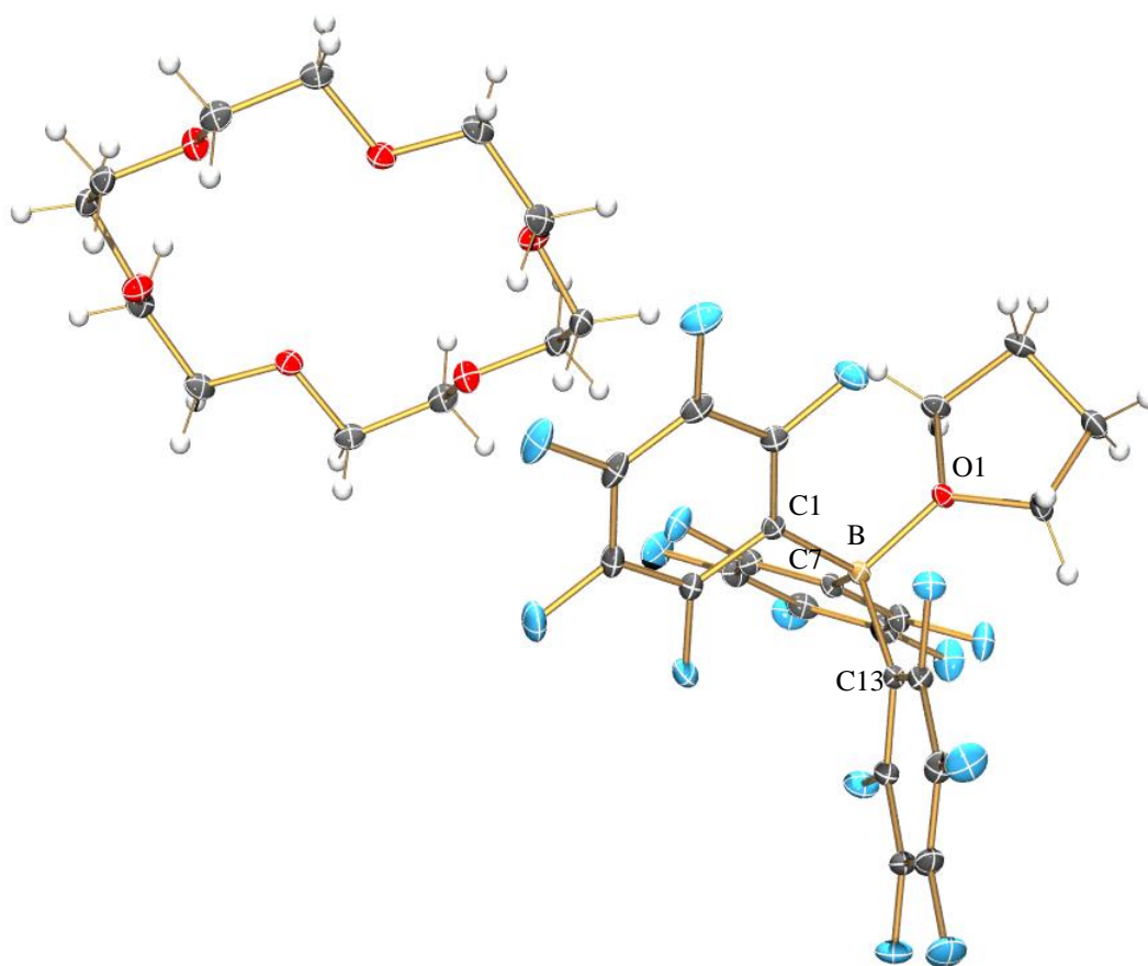
Abbildung 39. ORTEP-Darstellung der Molekülstruktur von (18-Krone-6) [THF·B(C 6 F 5 ) 3 ] auskristallisiert mit 18-Krone-6. Thermische Ellipsoide entsprechen 50% Wahrscheinlichkeit bei 173 K. Ausgewählte Abstände (Å) und Winkel (°): O1–B 1.572(1), B–C7 1.638(1), B–C13 1.640(1), B–C1 1.643(1), C1–C2 1.383(1), C1–C6 1.398(1), C2–C3 1.394(1), C3–C4 1.373(2), C4–C5 1.374(2), C5–C6 1.382(1), O1–B–C7 109.63(7), O1–B–C13 103.27(7), O1–B–C1 109.26(7), C7–B–C13 114.87(7), C7–B–C1 105.18(7), C13–B–C1 114.57(7), O1–B–C1–C2 6.8(1), C7–B–C1–C2 110.8(1), C13–B–C1–C2 122.1(1), O1–B–C1–C6 179.61(7), C7–B–C1–C6 62.0(1), C13–B–C1–C6 65.1(1).
