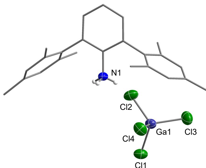
Abbildung 31. ORTEP-Darstellung der Molekülstruktur von [\text{TerNH}_3][\text{GaCl}_4] im Kristall. Zur Übersichtlichkeit sind die Wasserstoffatome, mit Ausnahme der NH-Protonen, ausgespart. Thermische Ellipsoide sind mit 50 % Wahrscheinlichkeit bei 173 K abgebildet.
