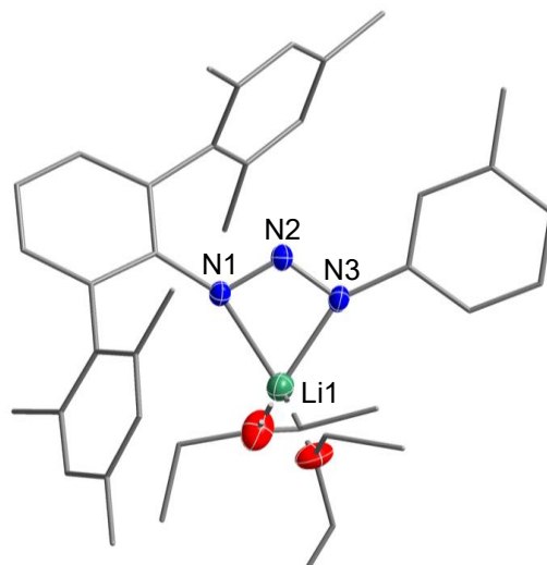
Abbildung 4. ORTEP-Darstellung der Molekülstruktur des Lithium-Triazenidsalzes 2TerTol im Kristall. Thermische Ellipsoide sind mit 50 % Wahrscheinlichkeit bei 173 K abgebildet. Ausgewählte Abstände (Å) und Winkel (°): Li1–N1 2.120(3), Li1–N3 2.005(3), N1–N2 1.316(2), N2–N3 1.309 (2), N1–Li1–N3 62.46(9), N1–N2–N3 109.4(2), Li1–N1–N2–N3 –1.0(2).
