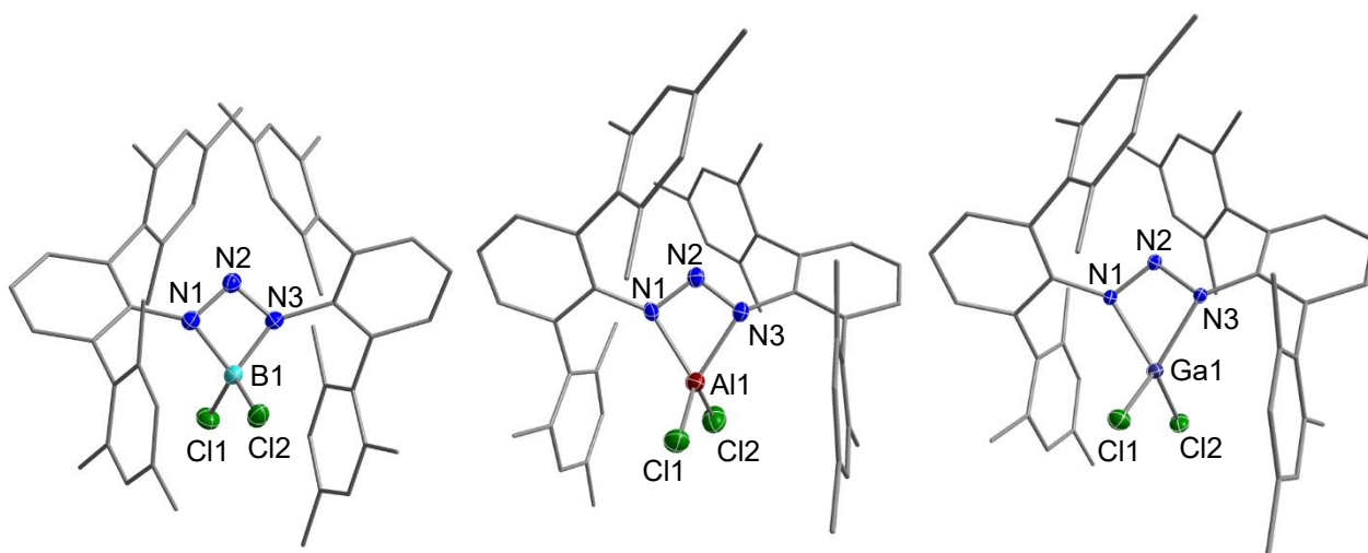
Abbildung 18. ORTEP-Darstellung der Molekülstruktur von [N( \mu -NTer) 2 BCl 2 ] ( 10B ), [35] [N( \mu -NTer) 2 AlCl 2 ] ( 10Al ) [35] und [N( \mu -NTer) 2 GaCl 2 ] ( 10Ga ) im Kristall. Thermische Ellipsoide sind mit 50 % Wahrscheinlichkeit bei 173 K abgebildet. Ausgewählte Abstände und Winkel sind in Tabelle 5 zusammengefasst.
