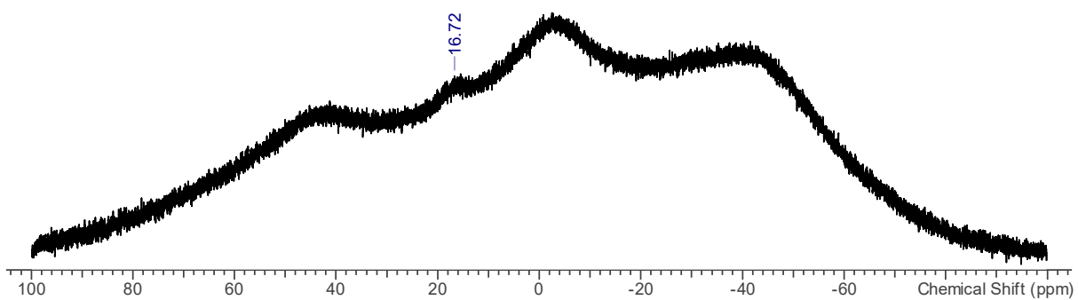
^{31}\text{P} -NMR-Spektrum
