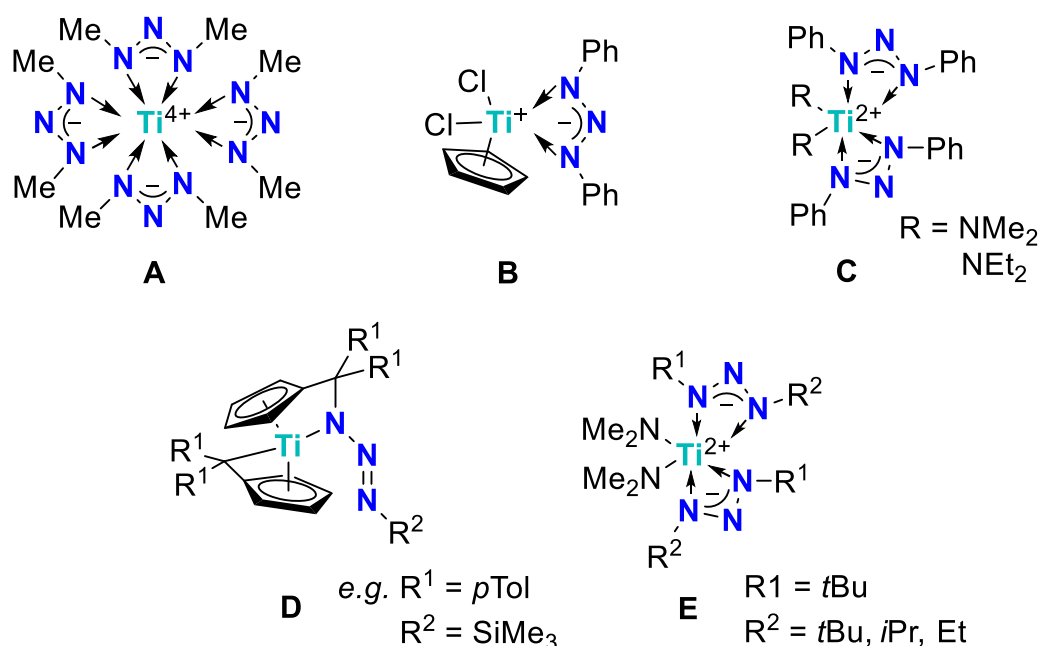
Abbildung 2. Bekannte Titan-Triazenido-Komplexe.
