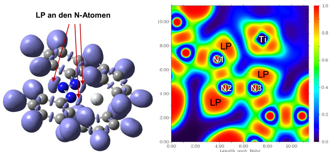
Abbildung 7. Links: ELF-Isofläche (iso = 0.90) von 3Ph . Rechts: 2D-Kontur-Plot der ELF.
