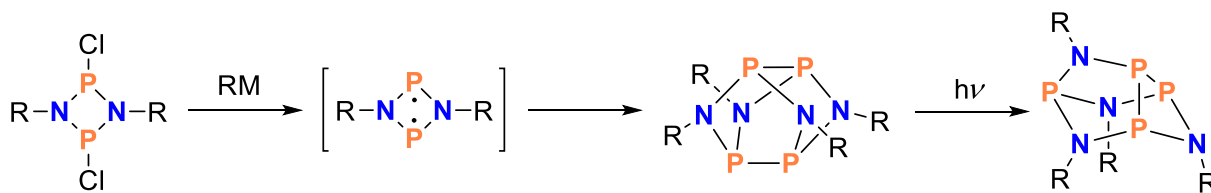
Abbildung 14. Mechanismus zur Bildung der \beta -Käfige ( \text{R} = t\text{Bu}, (\text{Me}_3\text{Si})_2\text{N}, \text{Dmp}, \text{Dipp} ).
