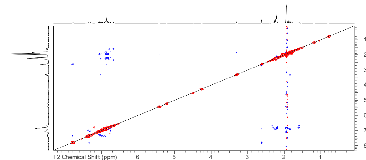
1 H- 1 H-NOESY-NMR-Spektrum
