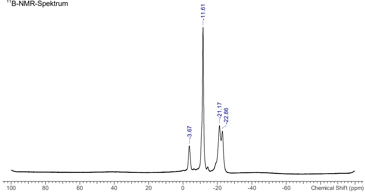
^{11}\text{B} -NMR-Spektrum
