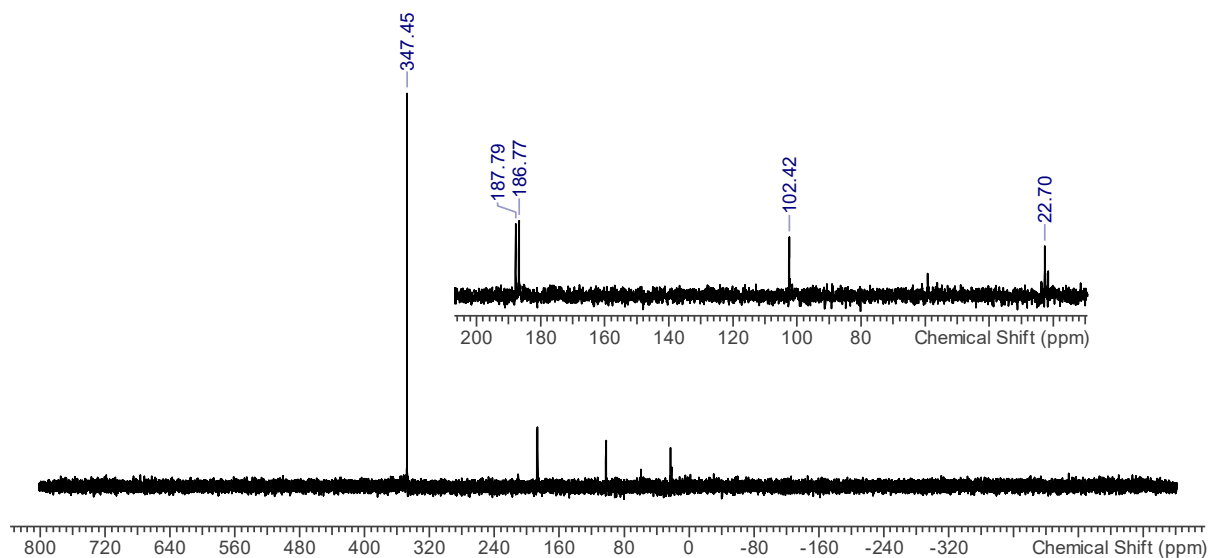
^{31}\text{P} -NMR-Spektrum
