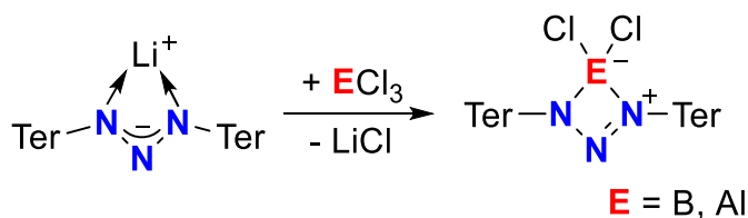
Schema 8. Synthese von Cyclobora- und -aluminatriazanen. [35]
