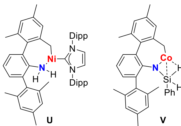
Abbildung 12. Bekannte, durch CH-Aktivierung der Terphenyl-Substituenten entstandene Übergangsmetallkomplexe.
