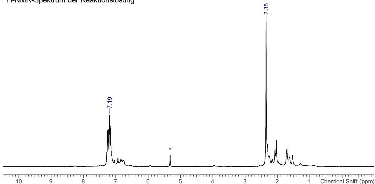
1 H-NMR-Spektrum der Reaktionslösung
