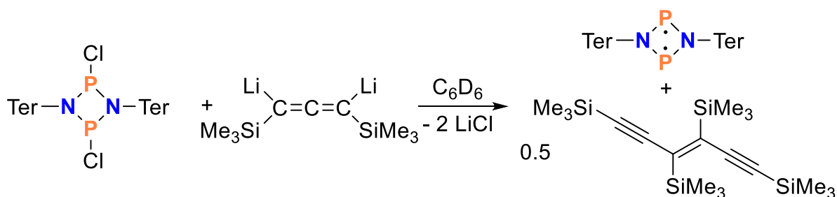
Schema 17. Reaktion von [\text{ClP}(\mu\text{-NTer})_2] mit \text{Li}_2[\text{Me}_3\text{SiC}_3\text{SiMe}_3] .
