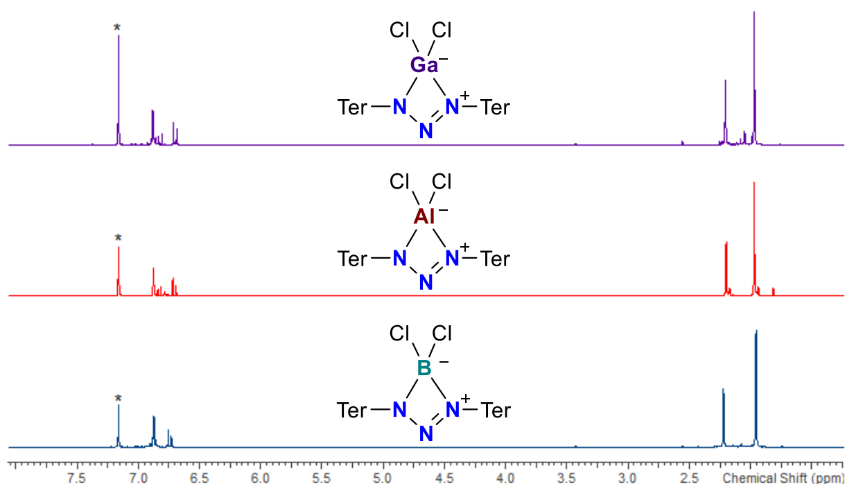
Abbildung 21. ^1\text{H} -NMR-Spektrum von 10B , 10Al und 10Ga (25 °C, ^*\text{C}_6\text{D}_6 , 300.13 MHz).
