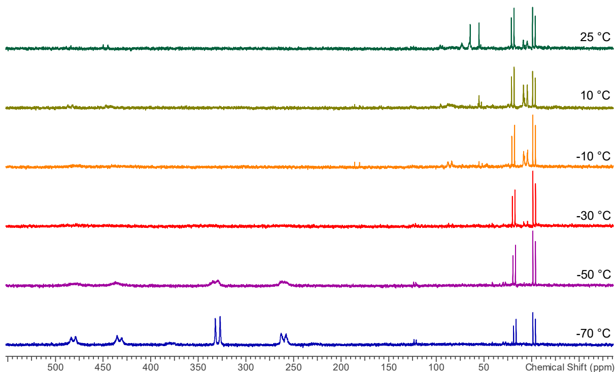
Abbildung 39. ^{31}\text{P} -NMR-Verfolgung der Tieftemperaturreaktion von \text{Mes}^*\text{PPN}(\text{BCl}_2)\text{Mes}^* ( 12 ) mit \text{GaCl}_3 von -70\text{ }^\circ\text{C} bis 25\text{ }^\circ\text{C} ( \text{CD}_2\text{Cl}_2 , 121.5 MHz).
