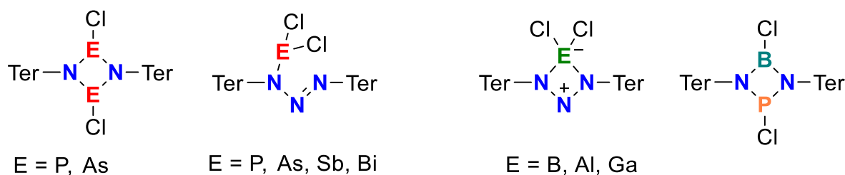
Abbildung 1. Bekannte Cyclopidniktadiazane und Cyclopniktatriazane (links) sowie die zu untersuchenden cyclischen Gruppe-13-triazane und das Cyclo-bora-phospha-diazan (rechts).
