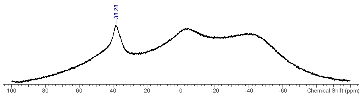
^{31}\text{P} -NMR-Verfolgung
