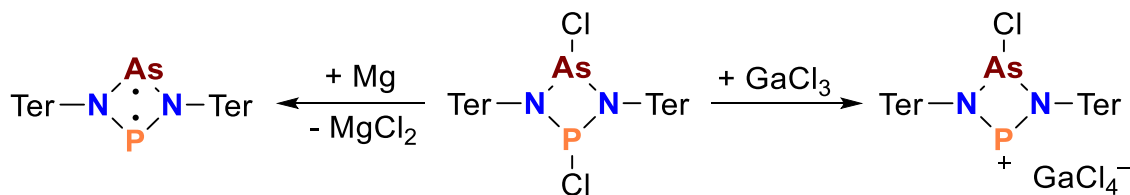
Schema 6. Reaktivität von [ClP(μ-NTer) 2 AsCl].
