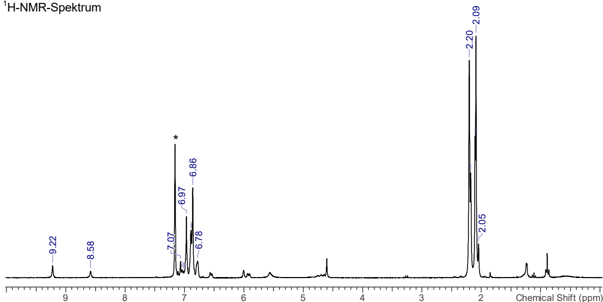
1 H-NMR-Spektrum
