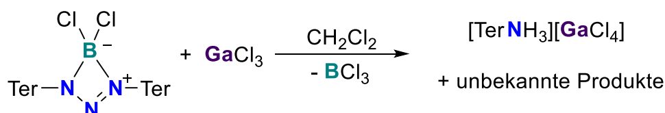
Schema 20. Reaktion von [\text{N}(\mu\text{-N}^+\text{Ter})_2\text{BCl}_2] ( 10B ) mit \text{GaCl}_3 in \text{CH}_2\text{Cl}_2 .
