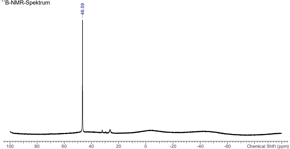
^{11}\text{B} -NMR-Spektrum
