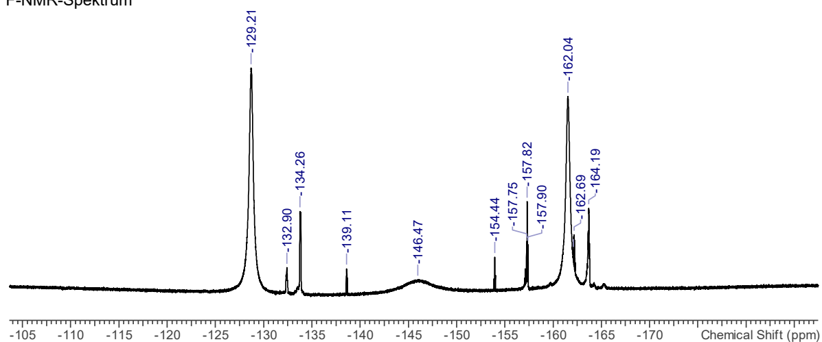
19 F-NMR-Spektrum
