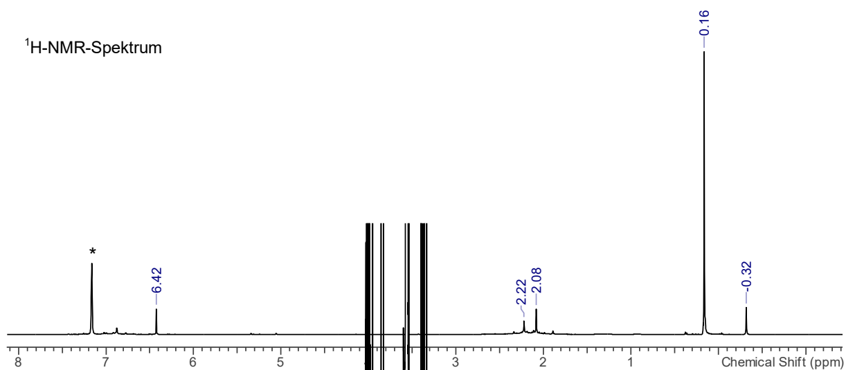
1 H-NMR-Spektrum
