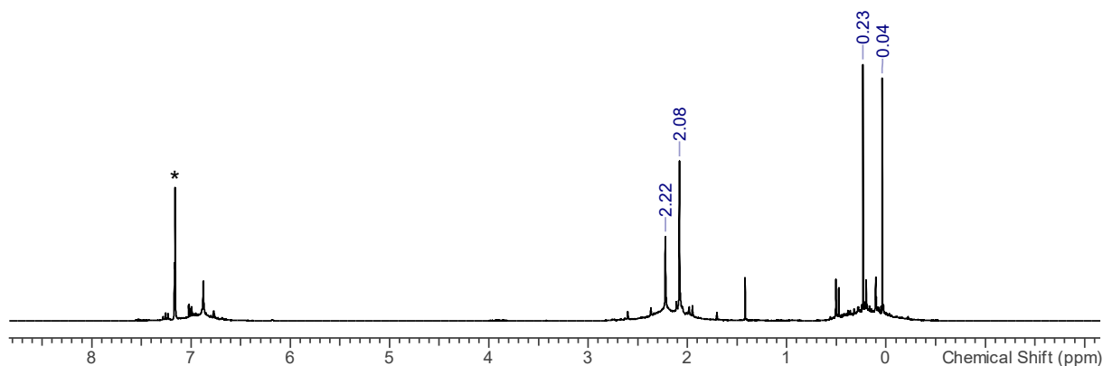
^1\text{H} -NMR-Spektrum
