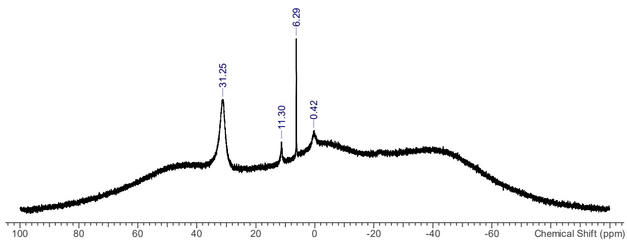
11 B-NMR-Spektrum
