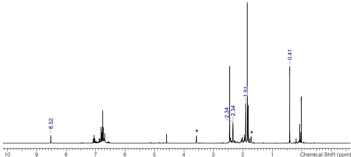
^1\text{H} -NMR-Spektrum
