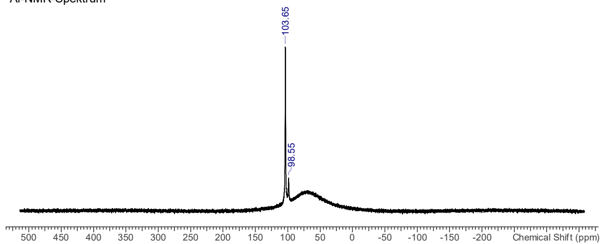
27 Al-NMR-Spektrum
