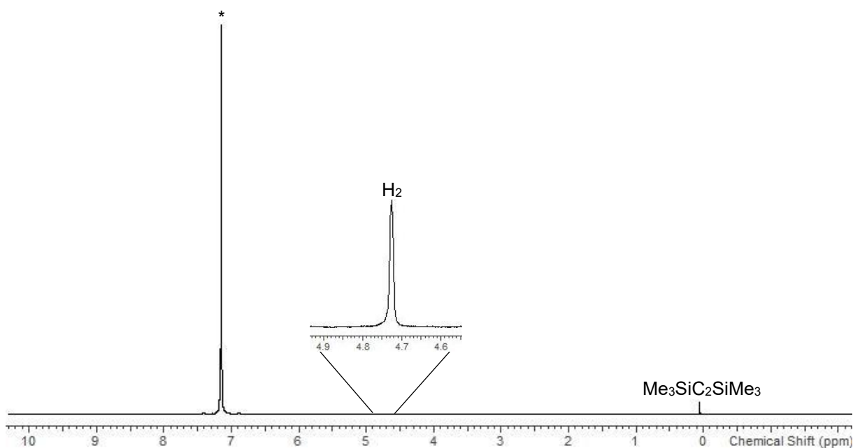
Abbildung 5. ^1\text{H} -NMR-Spektrum der Reaktionslösung von 1Ph mit \text{Cp}_2\text{Ti}(\eta^2\text{-Me}_3\text{SiC}_2\text{SiMe}_3) (25 °C, ^*\text{C}_6\text{D}_6 , 300.13 MHz).
