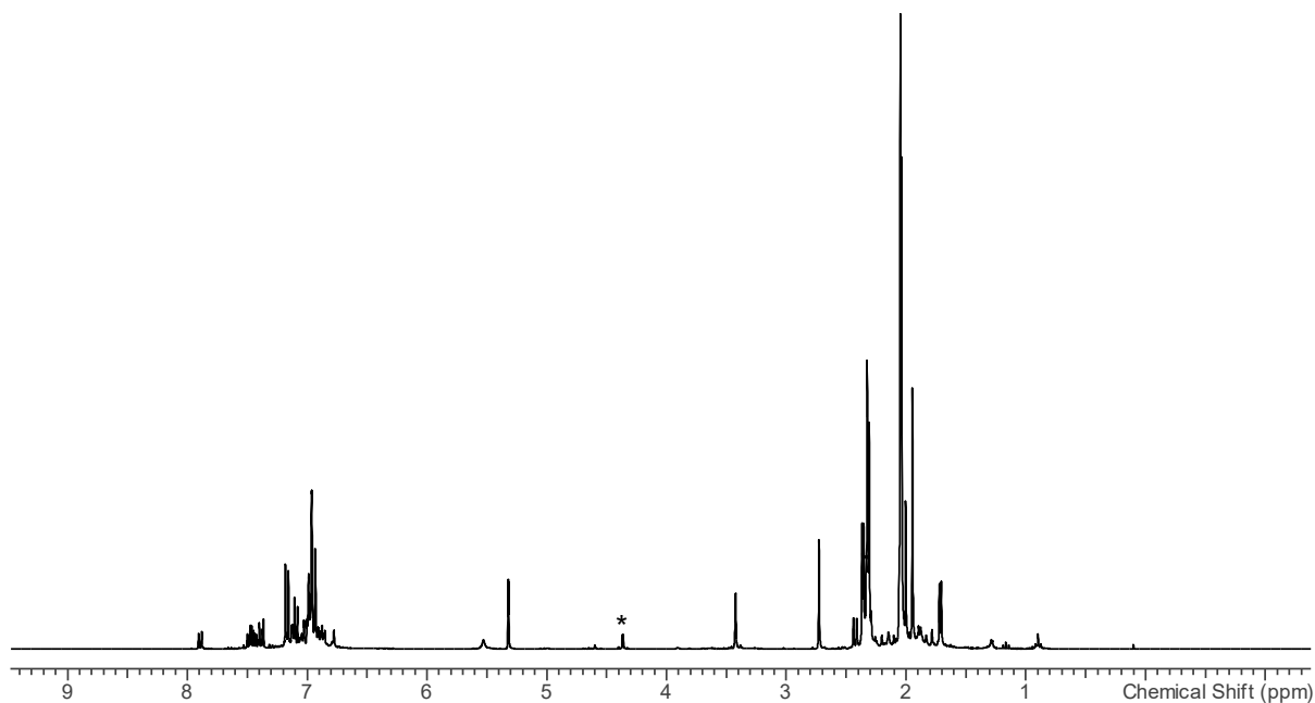
^1\text{H} -NMR-Spektrum
