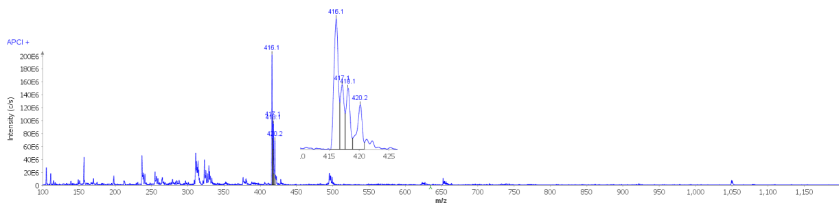
Abbildung 17. Massenspektrum (APCI ^+ ) des amorphen Produkts aus der Reaktion von \text{Cp}_2\text{Zr}(\text{py})(\eta^2\text{-Me}_3\text{SiC}_2\text{SiMe}_3) und 1Ph .
