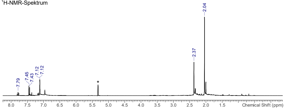
1 H-NMR-Spektrum
