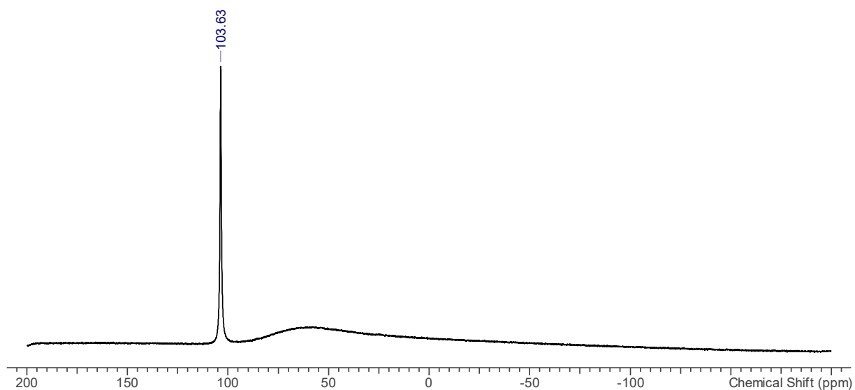
^{27}\text{Al} -NMR-Spektrum
