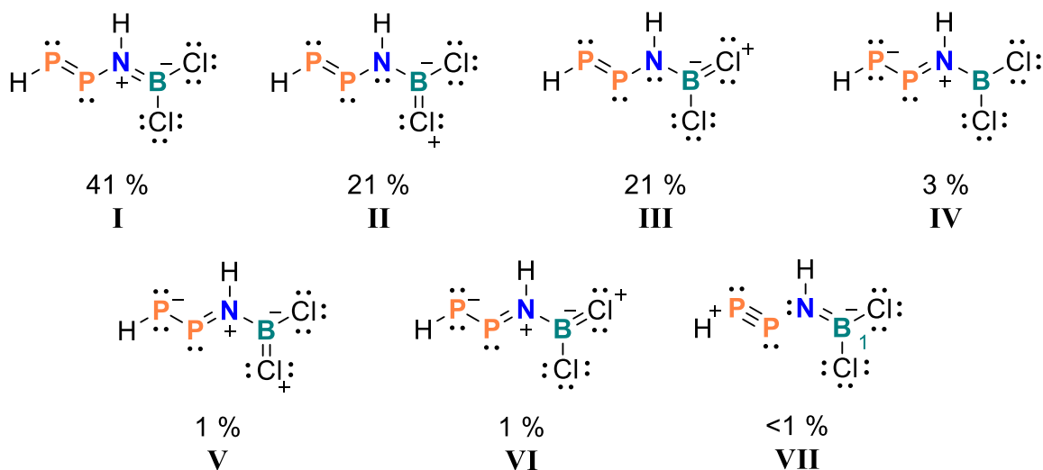
Abbildung 36. NRT-Resonanzschema von 12 mit Wasserstoff-Atomen.
