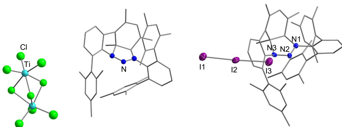
Abbildung 9. Konnektivität im Triazeniumsalz 5 (links) und ORTEP-Zeichnung der Molekülstruktur von 6 im Kristall (rechts). Thermische Ellipsoide mit 50 % Wahrscheinlichkeit bei 173 K. Ausgewählte Abstände (Å) und Winkel (°) von 6 : N1–N2 1.270(8), N2–N3 1.331(7), N1–C44 1.519(8), N3–C45 1.526(9), C44–C45 1.502(9), N1–N2–N3 109.5(5).
