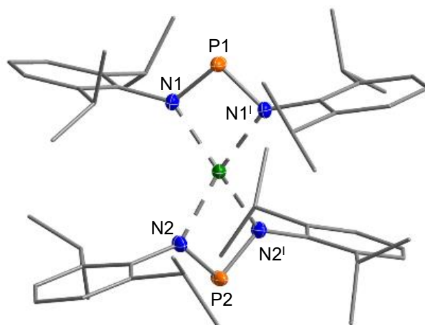
Abbildung 15. ORTEP-Darstellung der Molekülstruktur von 7 im Kristall. Thermische Ellipsoide sind mit 50 % Wahrscheinlichkeit bei 173 K abgebildet. Symmetry code: 2-x, y, 3/2-z. Ausgewählte Abstände (Å) und Winkel (°): N1–P1 1.608(1), N2–P2 1.605(1), N1–Mg1 2.056(1), N2–Mg1 2.053(1), N1–P1–N1' 98.8(1), N2–P1–N2' 98.6(1), N1–Mg1–N1' 72.8(1), N2–Mg1–N2' 72.9(1).
