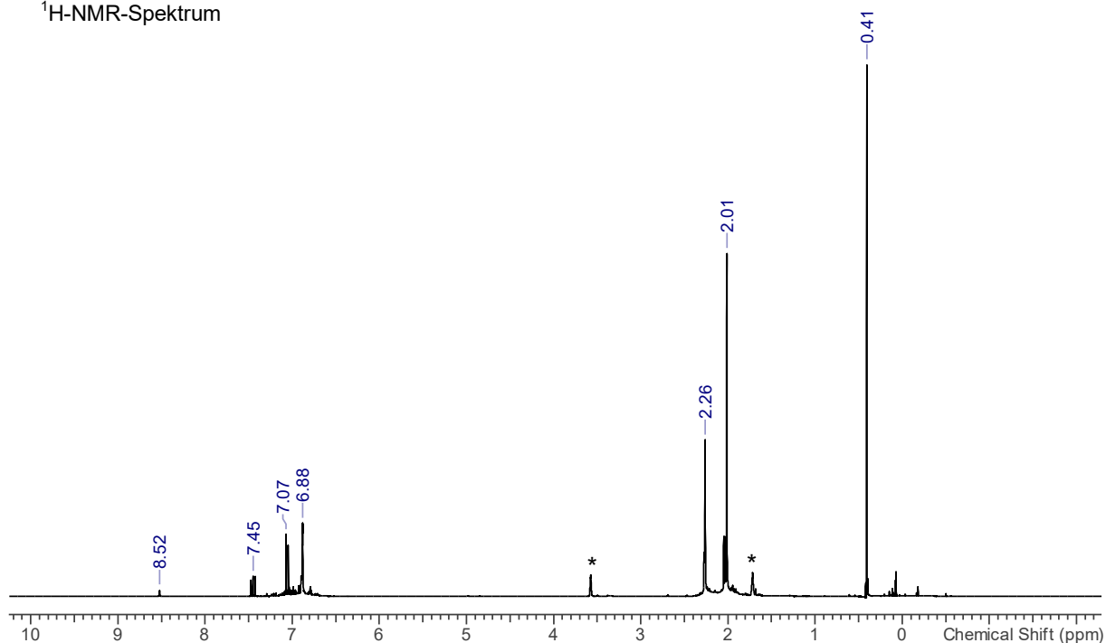
^1\text{H-NMR} -Spektrum
