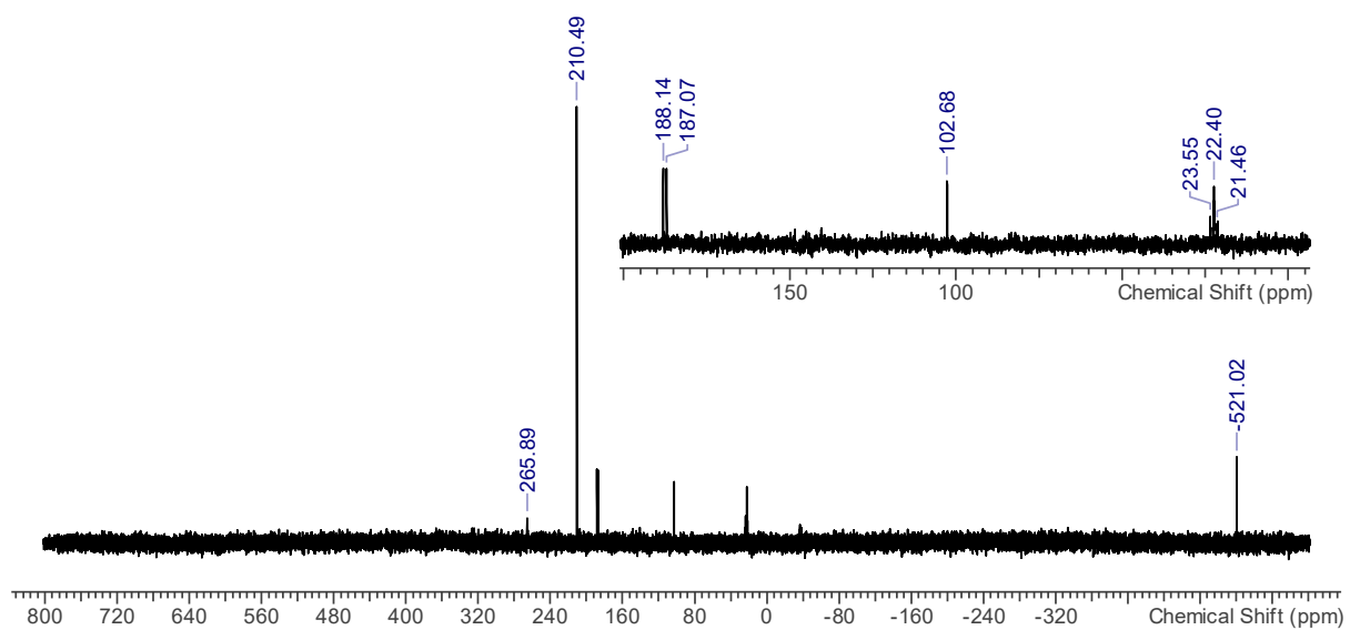
31 P-NMR-Spektrum
