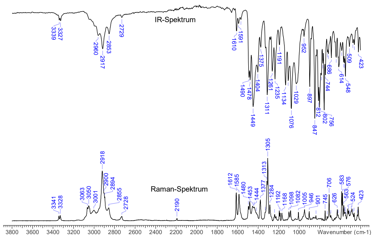
1 H-NMR-Spektrum
