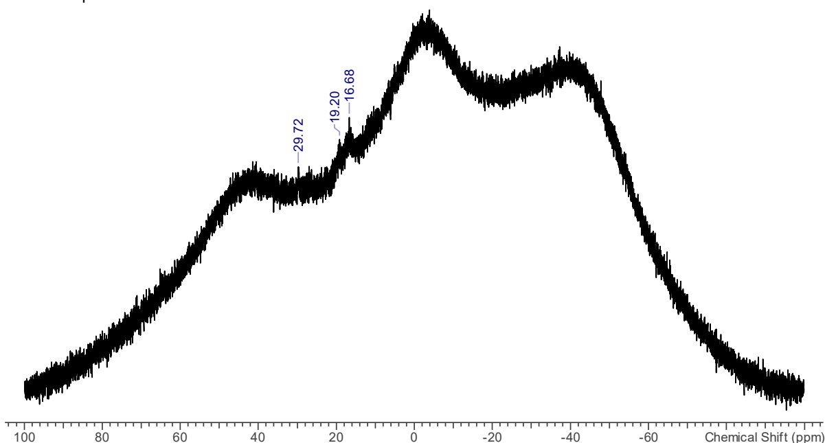
^{11}\text{B} -NMR-Spektrum
