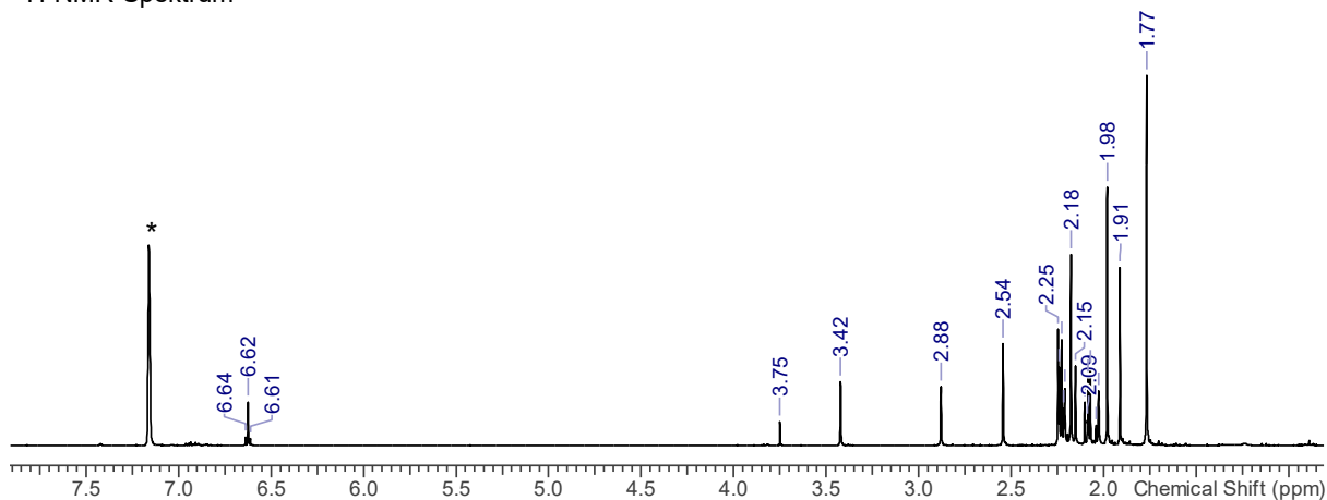
1 H-NMR-Spektrum
