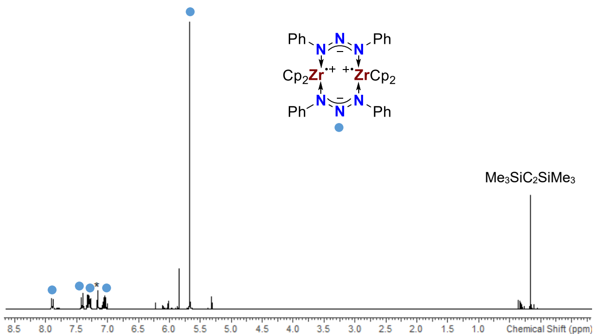
Abbildung 16. ^1\text{H} -NMR-Spektrum der Reaktionslösung von \text{Cp}_2\text{Zr}(\text{py})(\eta^2\text{-Me}_3\text{SiC}_2\text{SiMe}_3) mit \text{PhNNN}(\text{H})\text{Ph} 3Ph (25 °C, \text{C}_6\text{D}_6 , 300.13 MHz).
