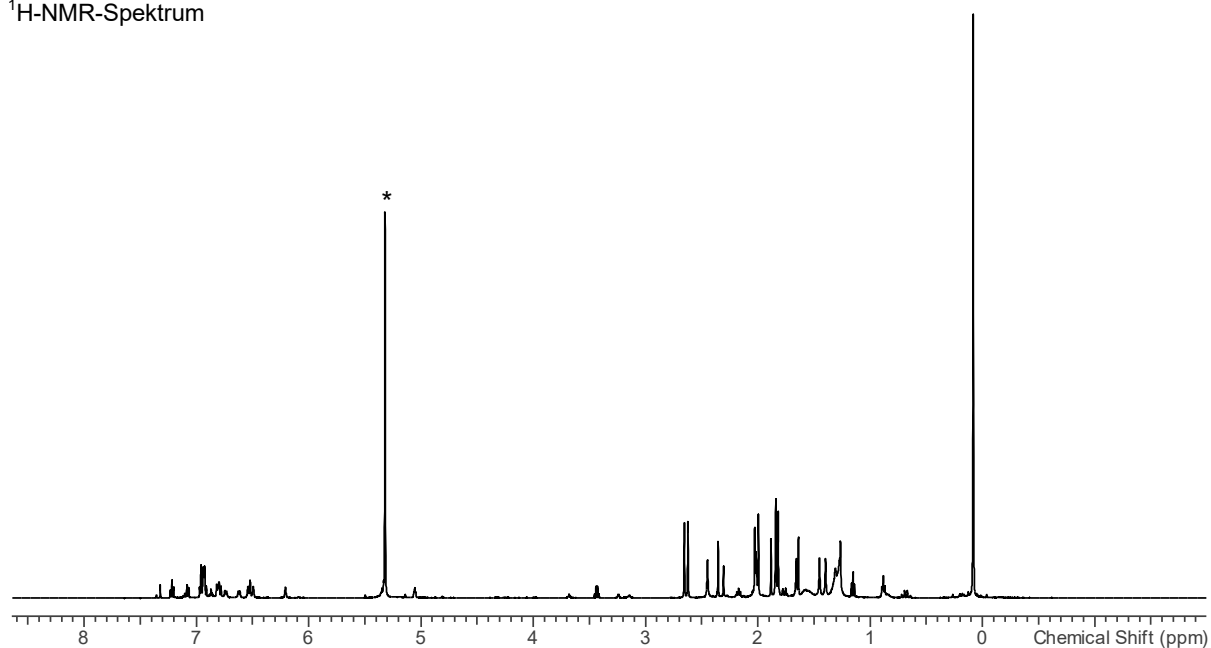
1 H-NMR-Spektrum
