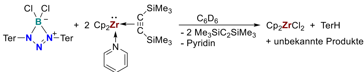
Schema 16. Reaktion von [\text{N}(\mu\text{-NTer})_2\text{BCl}_2] ( 10B ) mit \text{Cp}_2\text{Zr}(\text{py})(\eta^2\text{-Me}_3\text{SiC}_2\text{SiMe}_3) in Benzol.
