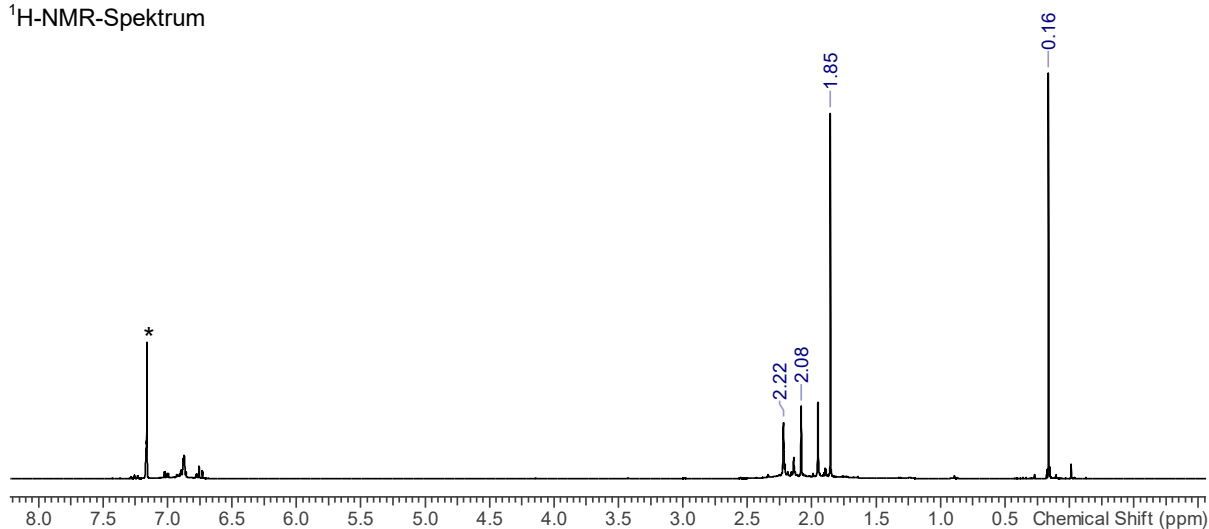
^1\text{H} -NMR-Spektrum
