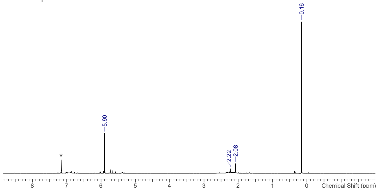
^1\text{H} -NMR-Spektrum
