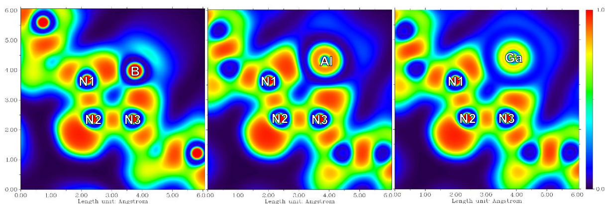
Abbildung 19. 2D-Kontur-Plots der ELF von 10B , 10Al und 10Ga .
