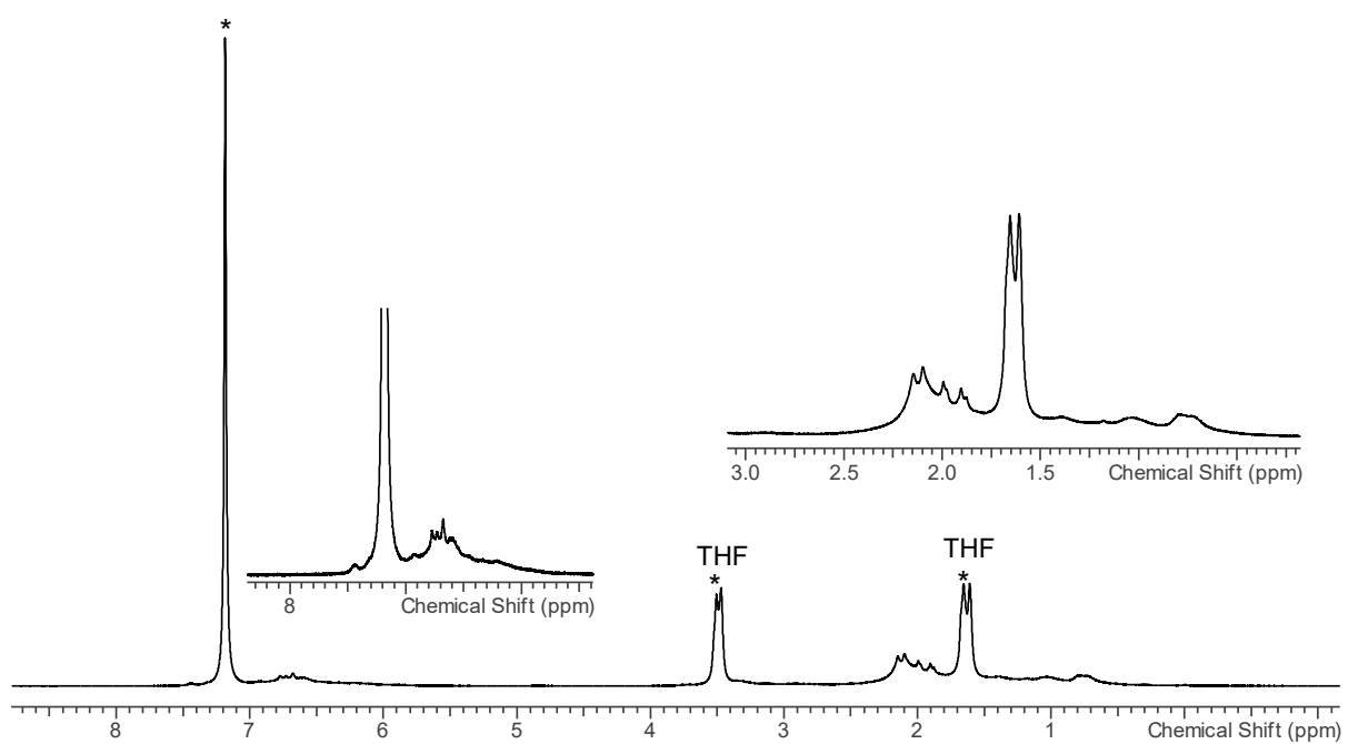
^1\text{H} -NMR-Spektrum in \text{THF-d}_8
