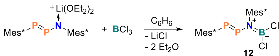
Schema 23. Synthese von Mes*PPN(BCl 2 )Mes* ( 12 ).
