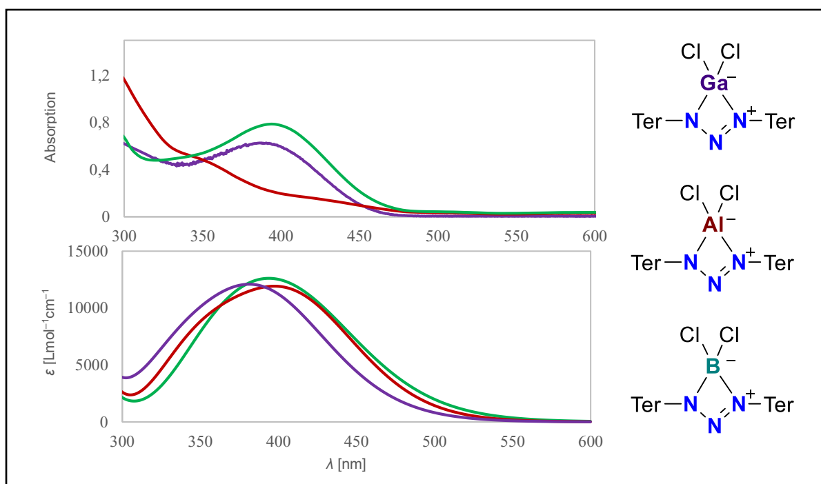
Abbildung 22. UV-Vis-Spektren von 10E (E = B, Al, Ga): experimentell in n -Hexan (oben), berechnet mit PBE-D3/def2-TZVP (unten).
