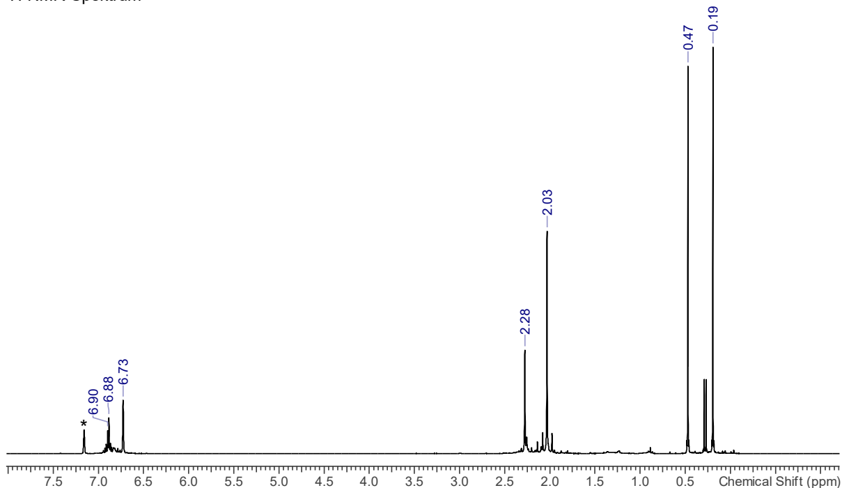
^1\text{H} -NMR-Spektrum
