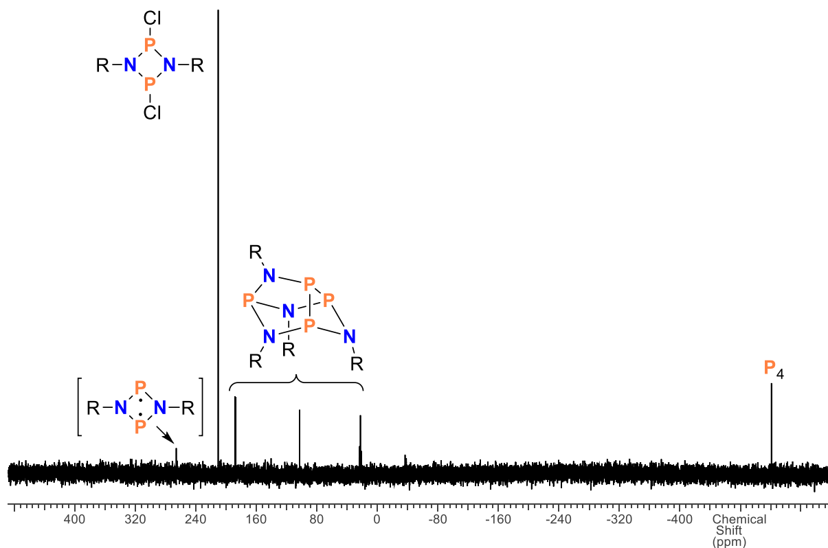
Abbildung 13. ^{31}\text{P} -NMR-Spektrum von [\text{ClP}(\mu\text{-NDipp})]_2 , \beta -Käfig [\text{PNDipp}]_4 und \text{P}_4 (25 °C, \text{C}_6\text{D}_6 , 300.13 MHz).
