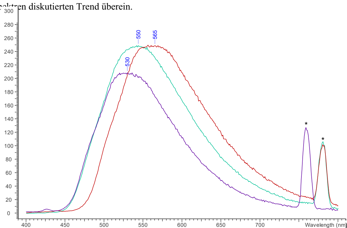
Abbildung 23. Fluoreszenz-Spektren von [\text{N}(\mu\text{-NTer})_2\text{BCl}_2] (grün, \lambda_{\text{ex}} = 390 nm), [\text{N}(\mu\text{-NTer})_2\text{AlCl}_2] (rot, \lambda_{\text{ex}} = 390 nm), [\text{N}(\mu\text{-NTer})_2\text{GaCl}_2] (violett, \lambda_{\text{ex}} = 380 nm) in n -Hexan. *Versuchsaufbau-bedingte Bande im Bereich der doppelten Anregungsfrequenz.
