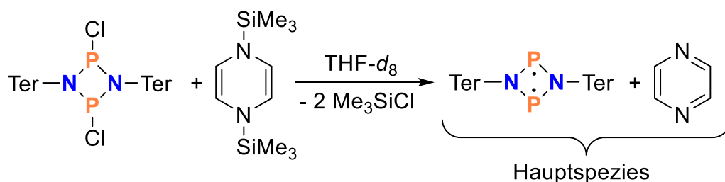
Schema 19. Reaktion von 1,4-Bis(trimethylsilyl)-pyrazin mit [\text{CIP}(\mu\text{-N}^{\text{Ter}})]_2 .
