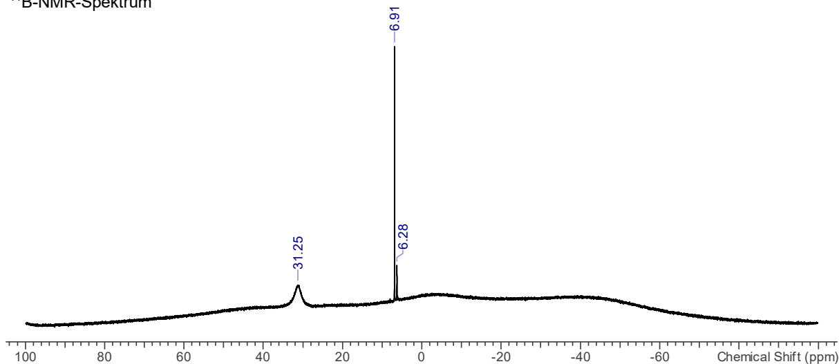
^{11}\text{B} -NMR-Spektrum
