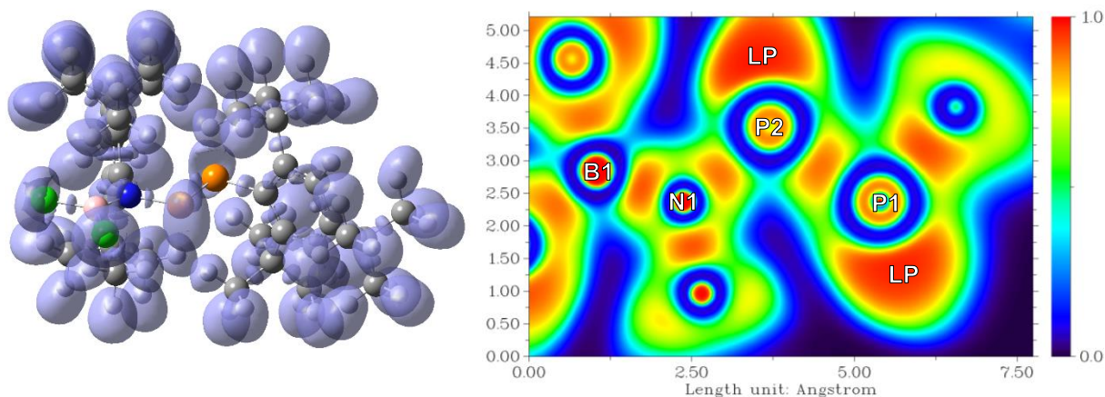
Abbildung 35. Links: ELF-Isofläche (iso = 0.85) von 12 . Rechts: 2D-Kontur-Plot der ELF.
