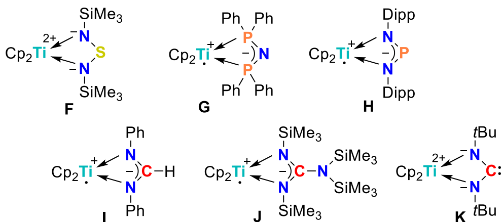
Abbildung 3. Darstellung von stickstoffhaltigen viergliedrigen Titanacyclen ausgehend von \text{Cp}_2\text{Ti}(\eta^2\text{-Me}_3\text{SiC}_2\text{SiMe}_3) und F : \text{Me}_3\text{SiSNSiMe}_3 , G : \text{Ph}_2\text{PN(H)PPh}_2 , H : [\text{DippNPCl}]_2 , I : \text{PhNC(H)N(H)Ph} , J : \text{Me}_3\text{SiNCNSiMe}_3 , K : t\text{BuNCN}t\text{Bu} . Es ist jeweils nur eine mögliche Strukturformel dargestellt.
