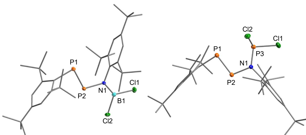
Abbildung 34. ORTEP-Darstellung der Molekülstruktur von Mes*PPN(BCl 2 )Mes* ( 12 ) und Mes*PPN(PCl 2 )Mes* [30] im Kristall. Thermische Ellipsoide sind mit 50 % Wahrscheinlichkeit bei 173 K abgebildet. Ausgewählte Abstände (Å) und Winkel (°) von 12 : B1–N1 1.404(2), B1–Cl1 1.765(2), B1–Cl2 1.762(2), N1–C19 1.458(2), N1–P2 1.749(1), P1–C1 1.873(1), P1–P2 2.034(1), N1–B1–Cl2 122.19(7), N1–B1–Cl1 121.66(7), B1–N1–P2 118.90(6), C1–P1–P2 91.05(3), N1–P2–P1 106.87(3) Cl1–B1–Cl2–N1 179.99(1).
