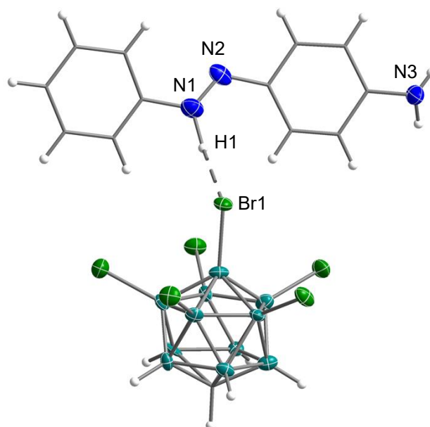
Abbildung 8. ORTEP-Zeichnung der Molekülstruktur von 4 im Kristall. Thermische Ellipsoide mit 50 % Wahrscheinlichkeit bei 173 K. Ausgewählte Abstände [Å]: N1–N2 1.257(8), H1–Br1 2.60(8).
