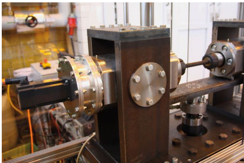
Entwickelter Umlaufbiegeprüfstand mit bis zu 3.000 rpm
