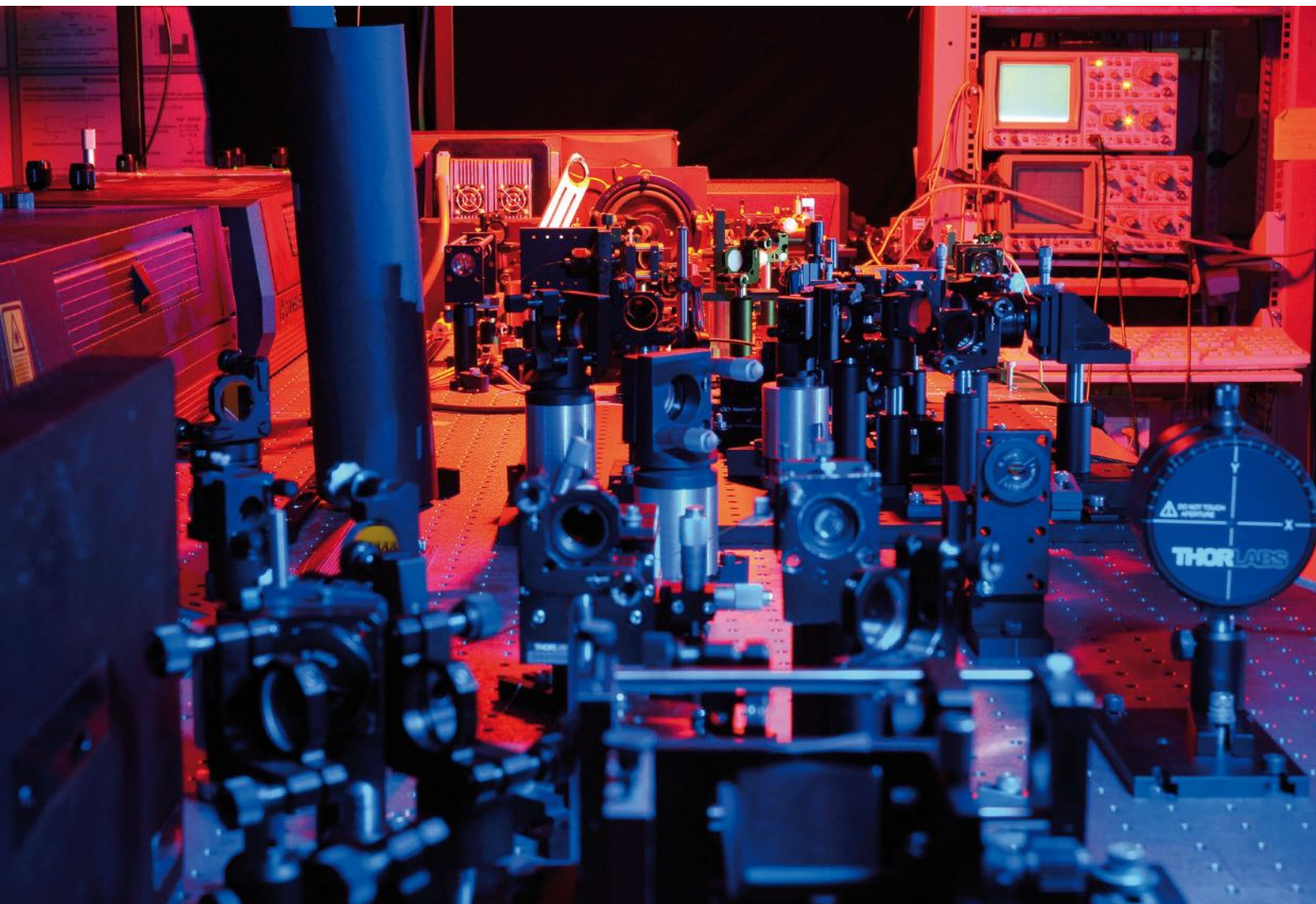
Experimenteller Aufbau zur Demonstration der Erhöhung der Datenrate in Glasfaserleitungen; Foto: F. Mitschke
