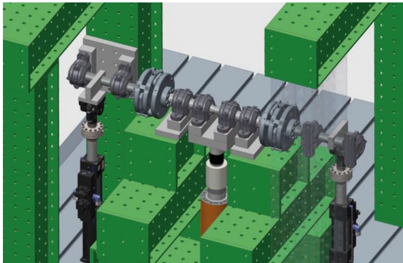
Konzept des Mixed-Mode-Prüfstandes, welches realisiert wird (CAD-Abbildung)
