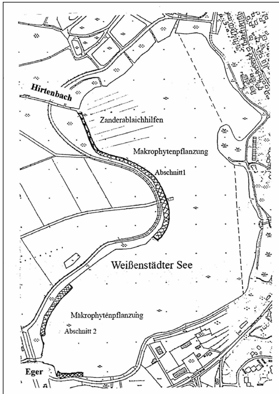
Abb. 1 Lage der bepflanzten Uferstreifen und Zanderablaichhilfen im Weissenstädter See
