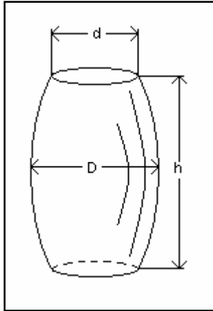
Abb. 3 Der als Modell für die Oosporenform benutzte parabolische Tonnenkörper
