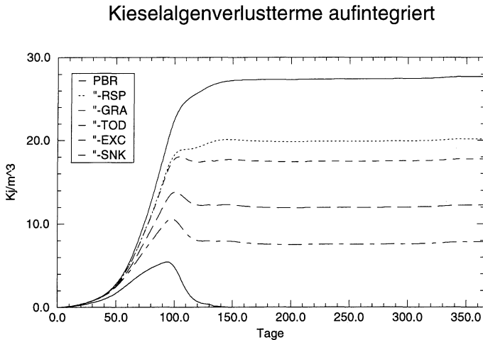
Abb. 18 Jahresgang der Produktions- und Verlustraten des Bacillariophyceen-Modelles, integriert
