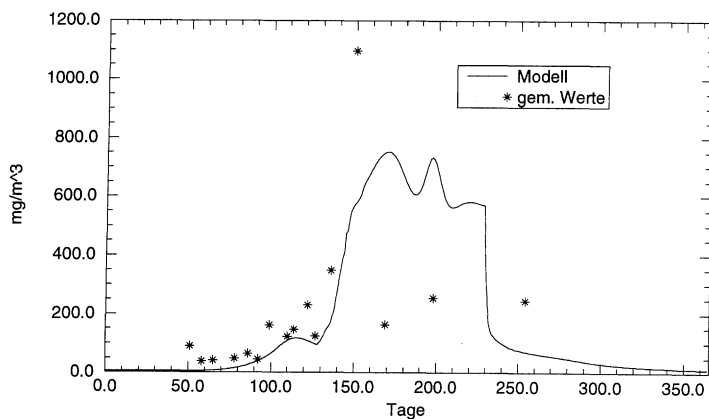
Abb. 11 Copepoda: Meßwerte und Modell 1989, Kompartiment Nordwesten (Meßwerte: BRENNING 1989)
